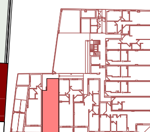
VIVIENDA B - PLANTA BAJA
