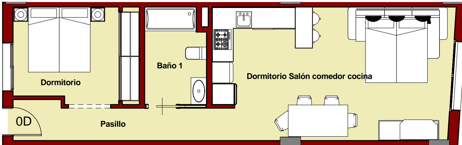
VIVIENDA D - PLANTA BAJA
