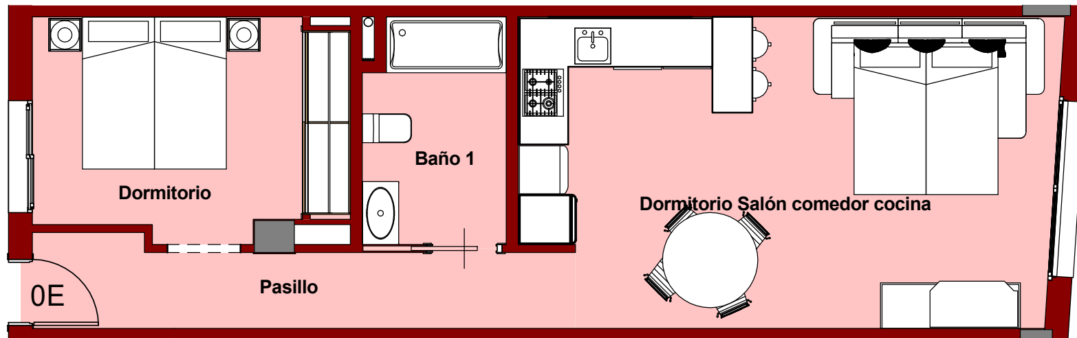
VIVIENDA E - PLANTA BAJA
