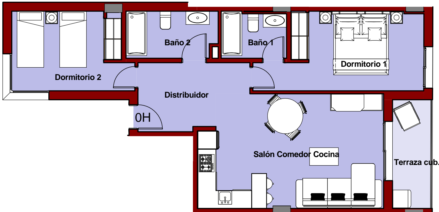
VIVIENDA H - PLANTA BAJA
