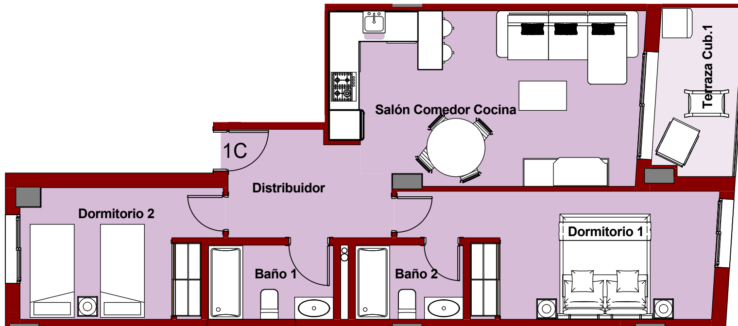
VIVIENDA C - PLANTA PRIMERA
