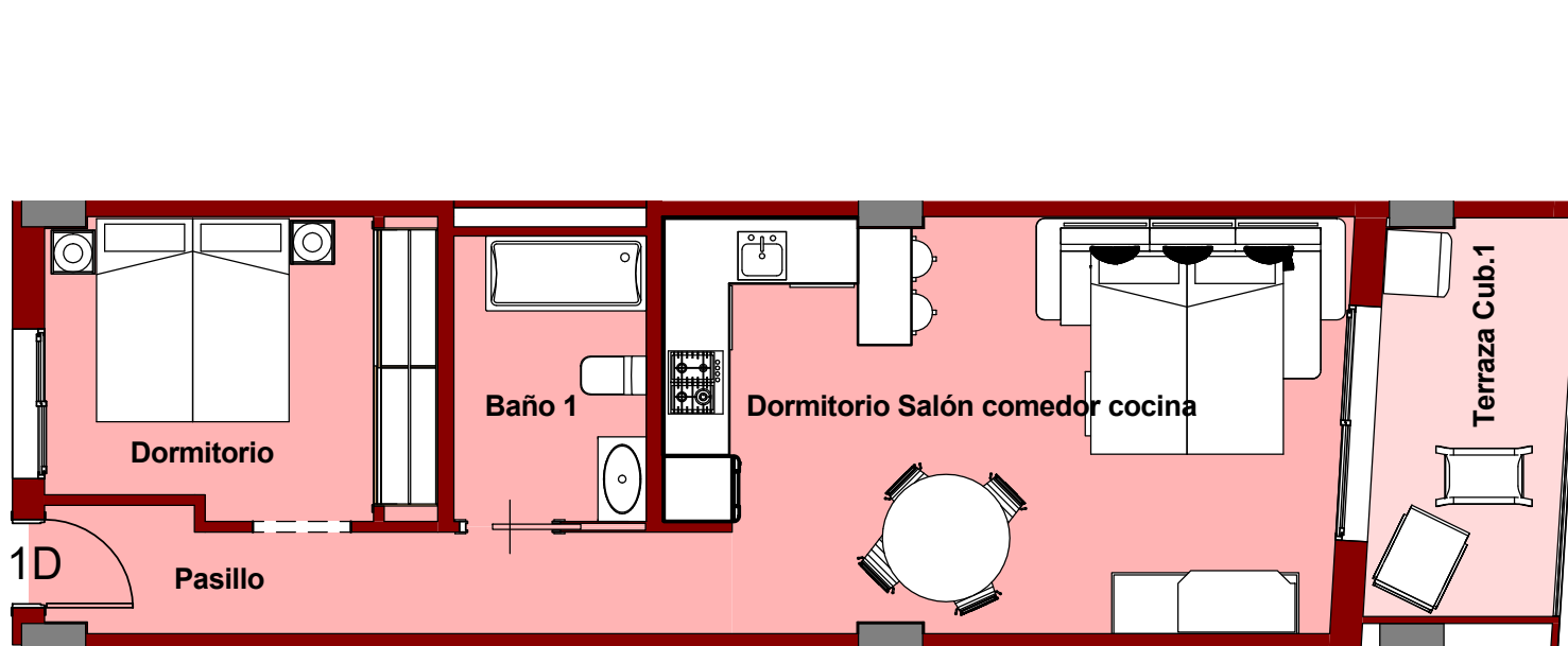
VIVIENDA D - PLANTA PRIMERA
