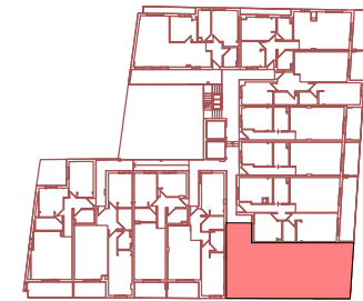
VIVIENDA G - PLANTA SEGUNDA
