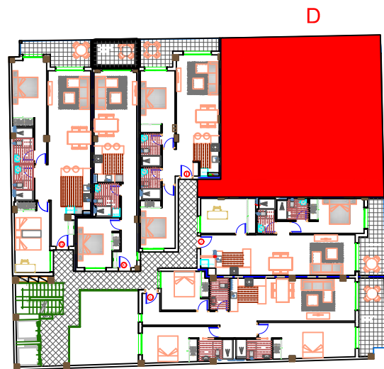
planta SEGUNDA
